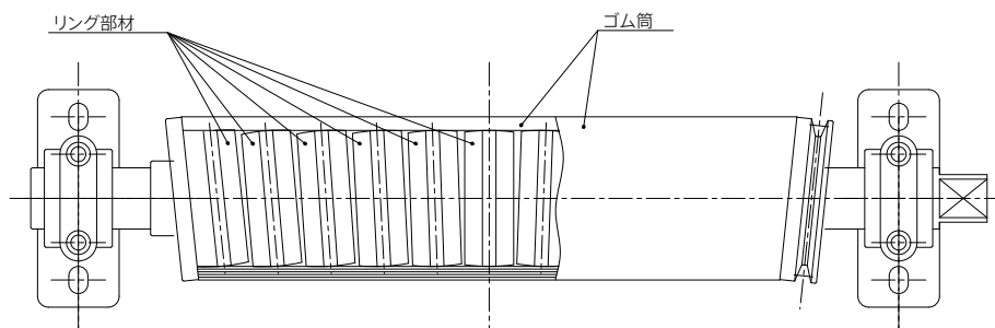
図2. MRV 構造
