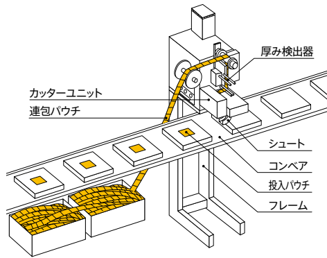
横ピロー包装機との接続
